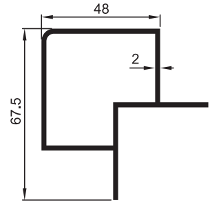
7008 1.255 kg/m 50'LİK 50 MM
