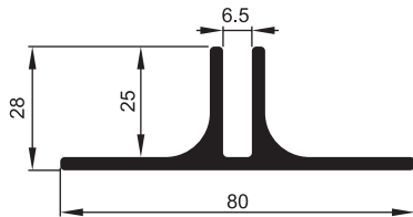
2115 B 1.225 kg/m Cam Bölme
