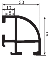
1121 A 0,486 gr/m Vitrin Köşe Profili
