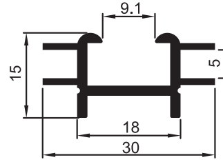
SM 1068 0.240 kg/m Aynasız Dikme
