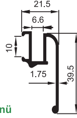
3108 0.485 kg/m Amortisörlü Cam Tutamağı
