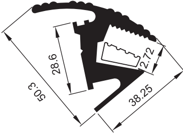
1107 B 1.573 kg/m Tırtırlı Amortisörlü Cam Kanalı
