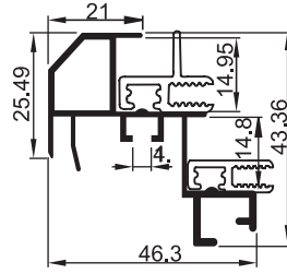
3125 H 0.600 kg/m Dondurma Dolabı Üst Sürgü Profili
