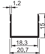
2105 G ( 1055 H ) 0.151 kg/m Sütlük Kenarı Isıcam "U" su
