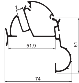
1118 B 1.185 kg/m Ön Küşpeşte
