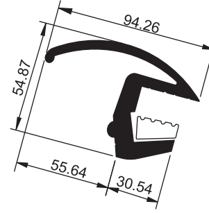
1107 C 3.250 kg/m Amortisörlü Cam Tutamağı
