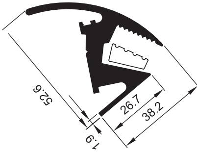
1107 A 1.620 kg/m Amortisörlü Cam Kanalı
