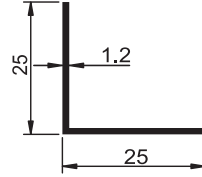
6119 A 0.167 kg/m Köşebent
