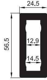
1113 A 2.239 kg/m Amortisör Kol Dikmesi
