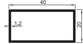
6118 A 0.393 kg/m Kutu Profil
