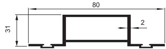
7012 1.000 kg/m Fitilli Orta Kayıt
