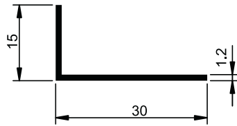
6119 D 0.150 kg/m Köşebent
