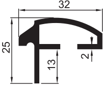
2116 0.409 kg/m Devirme Önü
