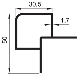
7010 0.735 kg/m 30'LUK 30 mm
