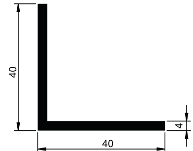
6119 M 0.655 kg/m Köşebent
