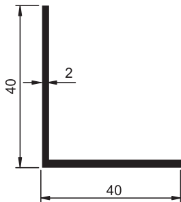
6119 H 0.443 kg/m Köşebent
