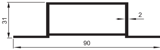
7011 1.100 kg/m Orta Kayıt
