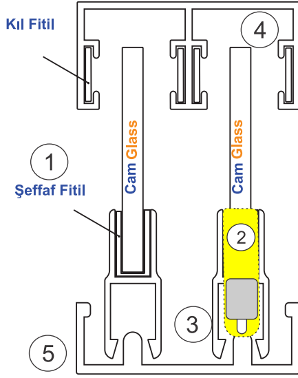
3 2110 A 0.245 kg/m Sürgü "H" ı
