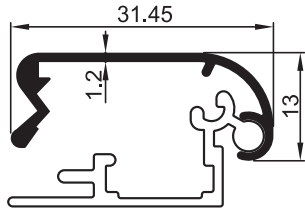
SM 1067 A 0.323 kg/m Kapı Çıtası
