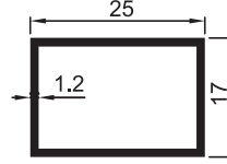
6118 0.270 kg/m Kutu Profil
