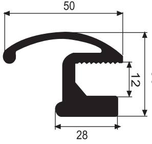
1107 D 1.175 kg/m Amortisörlü Cam Tutamağı
