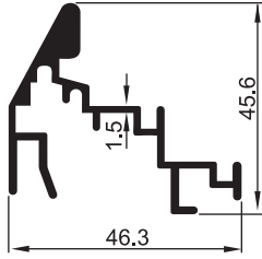
3125 0.885 kg/m Dondurma Dolabı Sürgülü Cam Kasası
