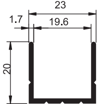
2105 F ( 1055 E ) 0.270 kg/m Sütlük Kenarı Isıcam "U" su
