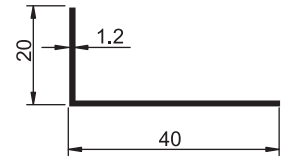
6119 C 0.200 kg/m Köşebent
