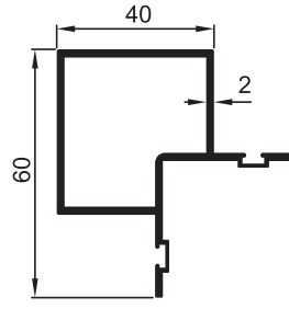
7009 1.090 kg/m 40'LİK 40 mm
