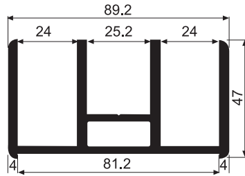
12690 2.746 kg/m Çiftli Kol Üstü Kovan Profili
