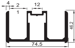
1117 2.492 kg/m Çiftli Kol Üstü
