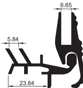
3111 A 0.685 kg/m Süslü Devirme Alt
