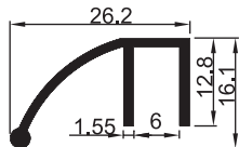
2106 A 0.230 kg/m Cam Tutacağı
