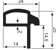
12655 0.421 kg/m Devirme Önü
