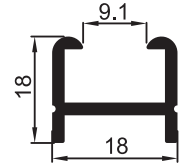
SM 1068 A 0.240 kg/m Aynalı Dikme
