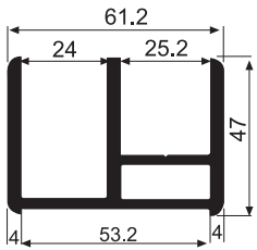
12656 2.066 kg/m Tekli Kol Üstü Kovan Profili
