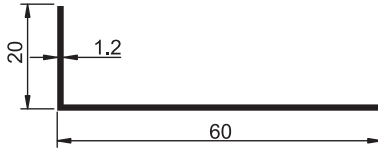
6119 0.270 kg/m 20x60 Köşebent
