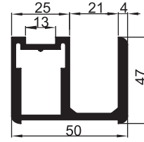
1113 A 2.239 kg/m Amortisör Kol Dikmesi
