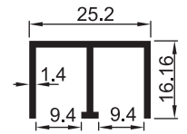
2112 0.355 kg/m Sürgü Rayı
