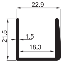
2115 A ( SM 1055 ) 0.330 kg/m Sütlük Kenarı Isıcam "U" su
