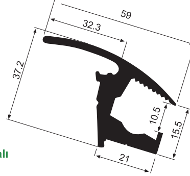
12677 1.288 kg/m Amortisörlü Cam Kanalı
