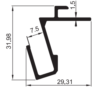
3128 0.370 kg/m Dondurma Dolabı Cam Profili
