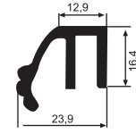
2106 D 0.378 gr/m Süslü Cam Tutamağı
