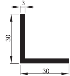
6119 G 0.485 kg/m 30x30X3mm. Köşebent
