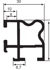
1121 A 0,486 gr/m Vitrin Köşe Profili
