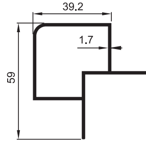
7007 0.900 kg/m 40'LİK 40 mm
