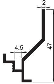
3125 A 0.390 kg/m Dondurma Dolabı Profili
