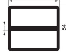
1112 2.730 kg/m Çift Amortisör Kol Dikmesi Çiftli Kutu
