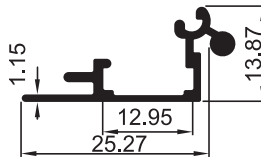
SM 1067 0.230 kg/m Görsel Çerçeve Profili
