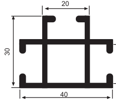
1121 D 0,549 gr/m Dekoratif Köşe
