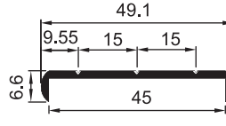
2105 B ( SM 1029 A ) 0.260 kg/m Çizgili Sütlük Kenarı 45 mm
