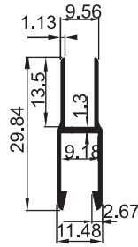
3 2110 A 0.245 kg/m Sürgü "H" ı
