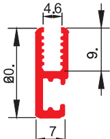
3125 G PVC Dondurma Dolabı Cam Çıtası
