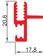
3125 J PVC Dondurma Dolabı Cam Çıtası
