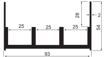
12676 2.298 kg/m Çiftli Kol Üstü Kovan Profili
